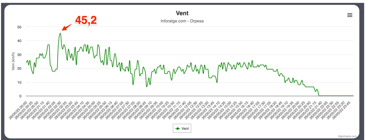
Ráfagas de viento registradas en OROPESA DEL MAR el 26/05/23 (en km/h) https://inforatge.com/meteo-oropesadelmar
